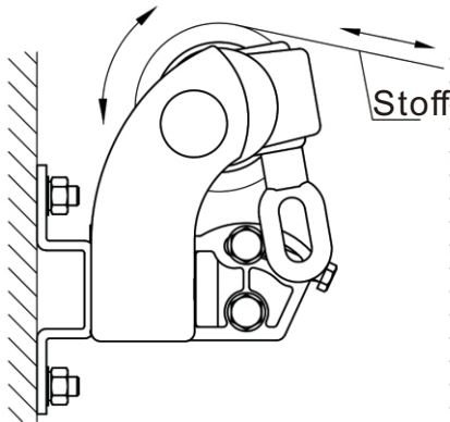
Richtige Bedienung
