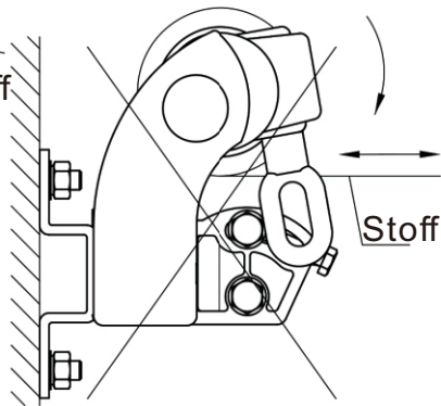
Falsche Bedienung
